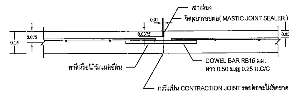
ขยายรอยต่อ CONTRACTION JOINT, CONTRACTION JOINT
